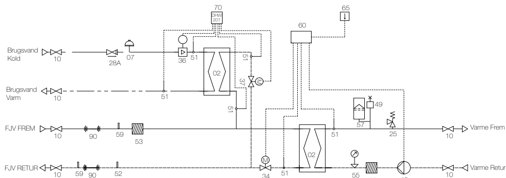
Principdiagram, Calefa V unit med ECL
