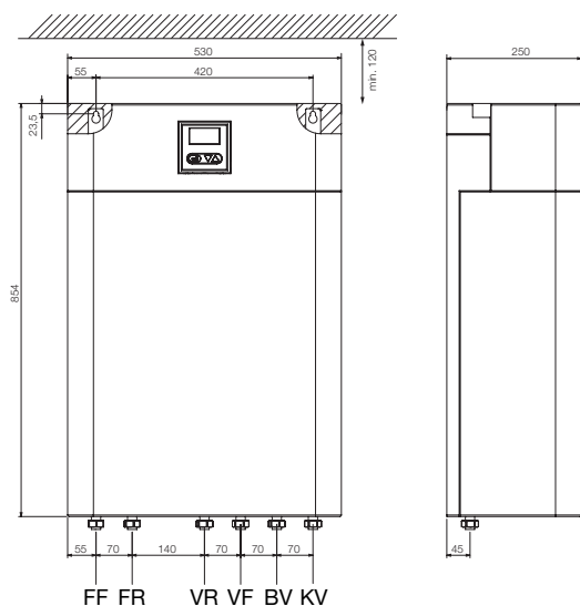
Tilslutningskitse, venstrevendt
