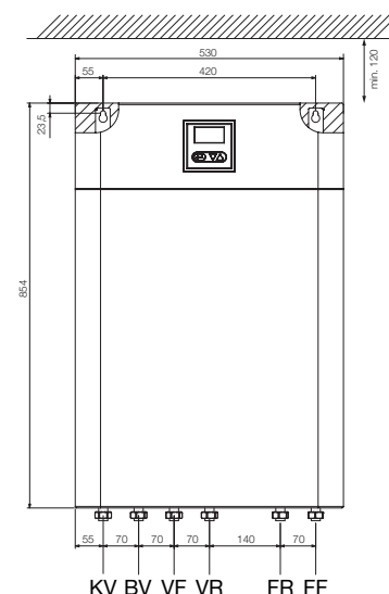
Tilslutningskitse, højrevendt
