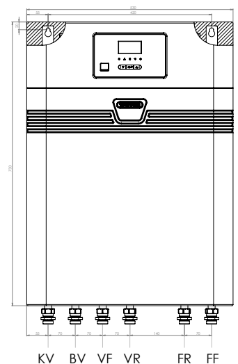
Tilslutningsskitse, højrevendt
